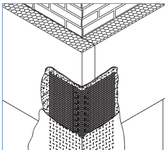
5 Ztužení nároží.
