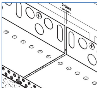
1b Vzájemné napojování zakládacích lišt.
