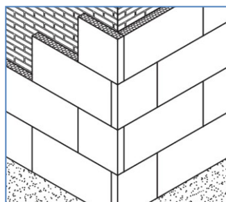
2c Lepení izolačních desek na nároží
