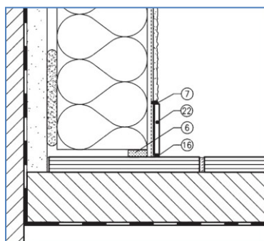
9c Ukončení ETICS u podlahy lodžie.
