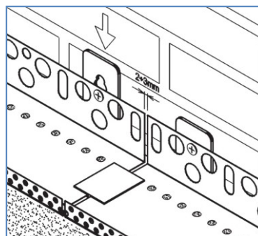
1c Vzájemné napojování zakládacích lišt., užití distančních podložek.
