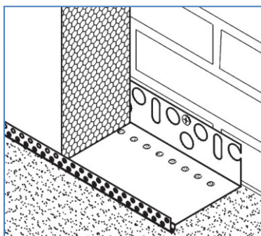
1a Založení první řady do zakládací lišty.
