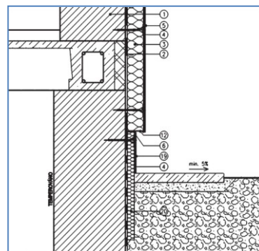
9b Ukončení ETICS pod terénem.
