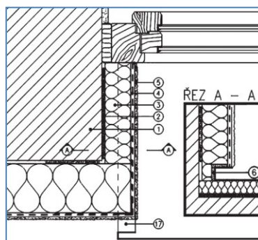
10b ETICS v oblasti přechodu ostění parapetu okna.
