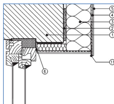
11a ETICS v oblasti okenního nadpraží.
