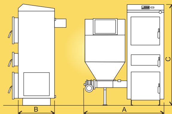
Schéma kotlů MASTER-M UNI
