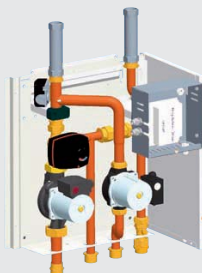
Sada pro připojení 2. topného okruhu
