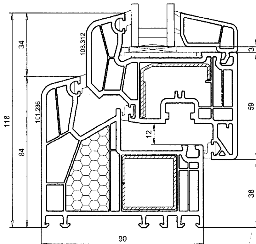
Obr. č. 1 Řez plastovým oknem – systém VEKA ALPHALINE 90
